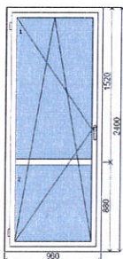
Balkónové dvere Vnútný pohľad (interiér)
